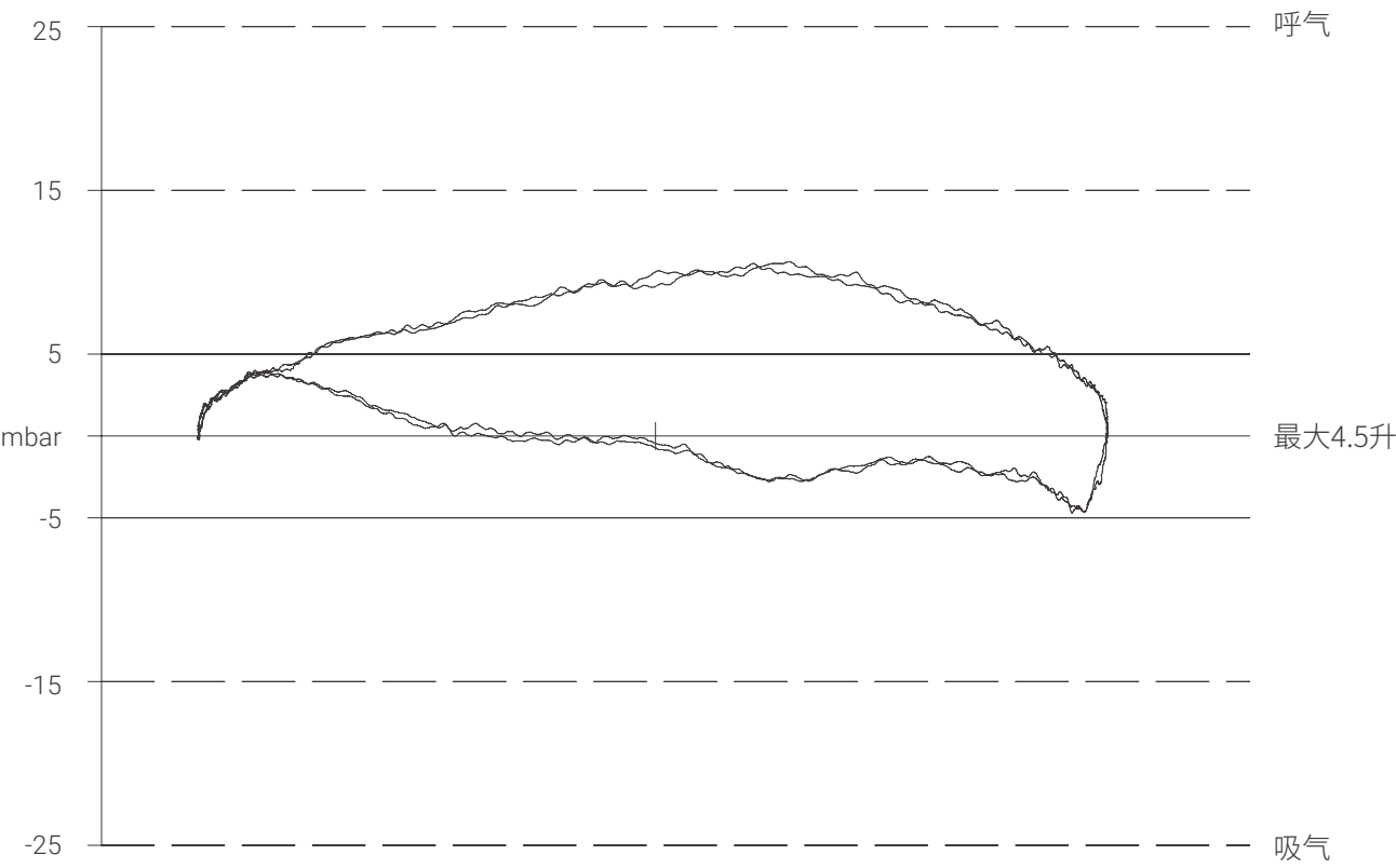
平均水深51.7 m (169.5 fsw)时的压力容积图
