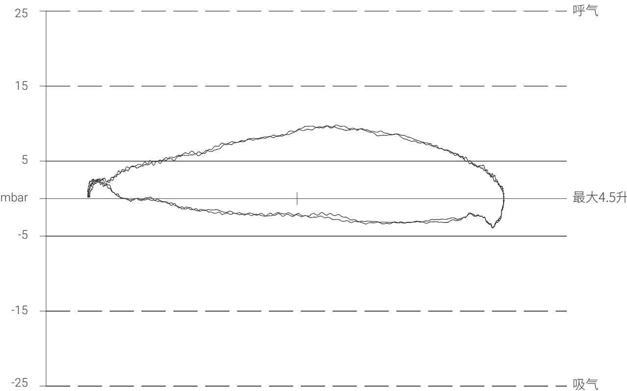
平均水深51.7 m (169.5 fsw)时的压力容积图
