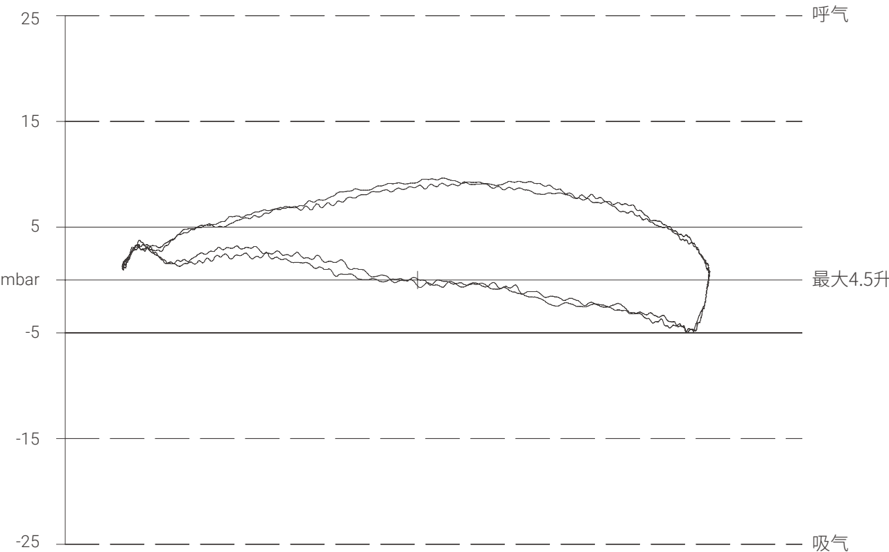
平均水深 51.9 m(170.4 fsw)时的压力容积图
