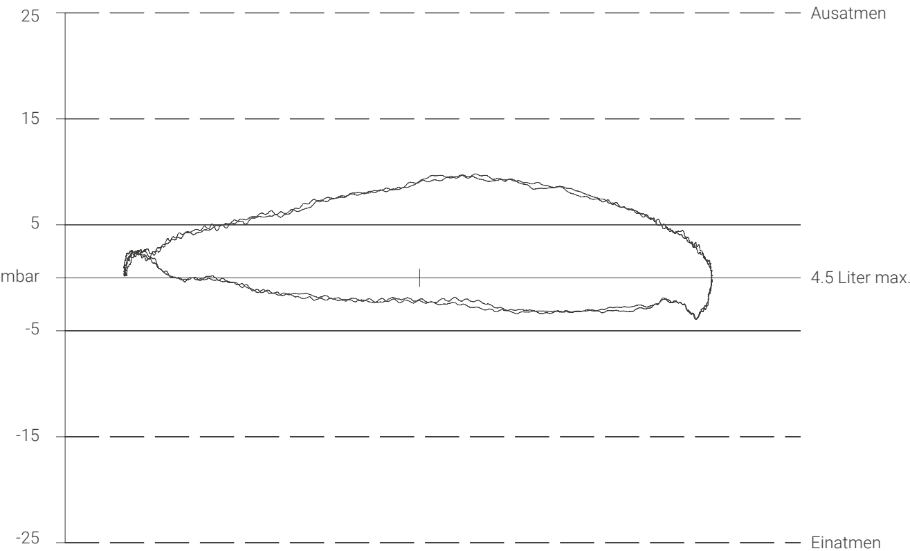
Druck-Volumen-Diagramm bei mittlerer Tiefe von: 51.7 msw (169.5 fsw)
