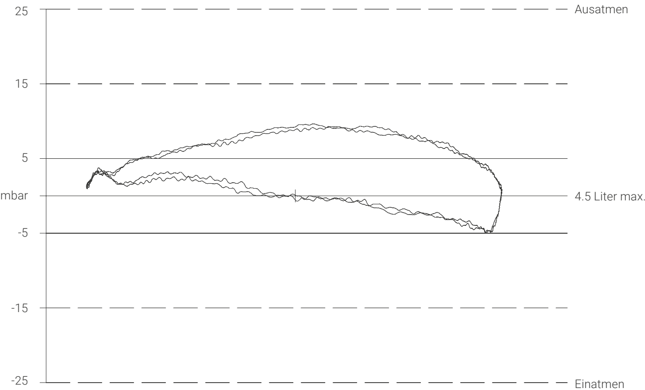
Druck-Volumen-Diagramm bei mittlerer Tiefe von: 51.9 msw (170.4 fsw)
